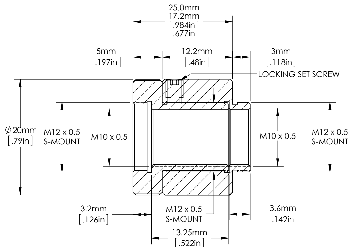
SECTION A-A
